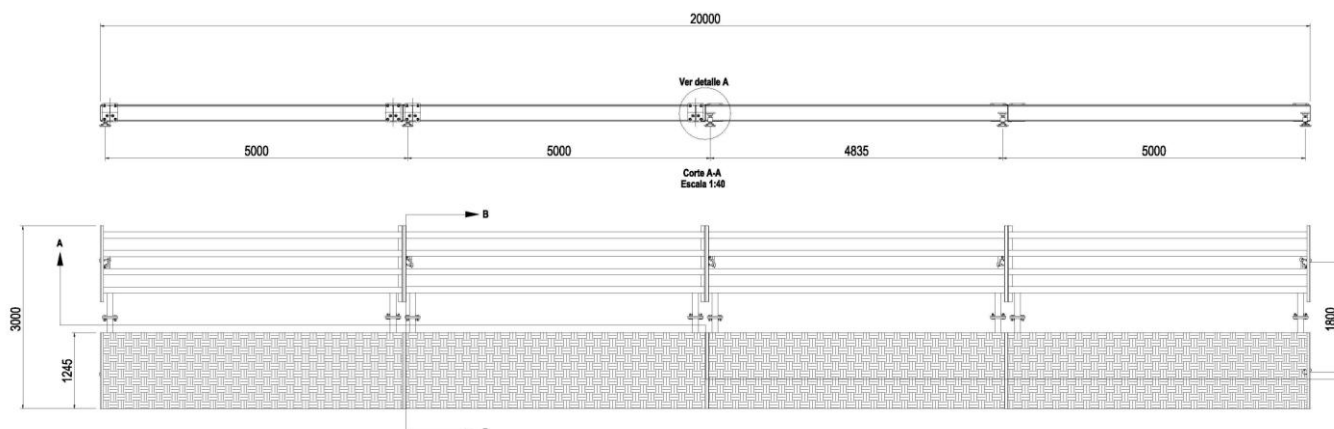
Dimensiones generales de una bascula largo 20 m
